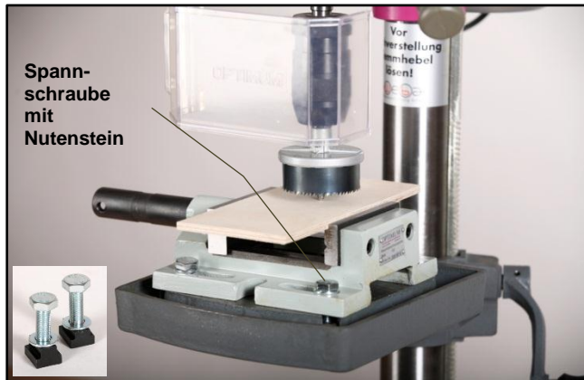
Bohren mit der Lochsäge: Festspannen des Schraubstockes auf dem Bohrmaschinentisch notwendig!
