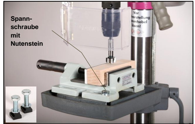
Große Bohrungen in große Werkstücke: Festspannen des Schraubstockes auf dem Bohrmaschinentisch notwendig!
